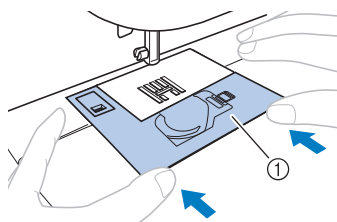
① Крышка игольной пластины
