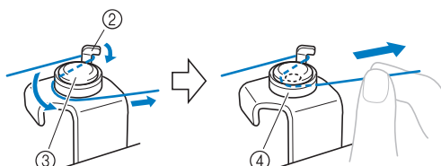
② Крючок ③ Диск предварительного натяжения ④ Протяните как можно дальше.
