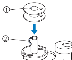
① Паз ② Пружина на валу устройства намотки шпульки
