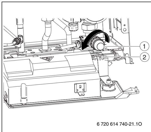
Рис 39 Предохранительный клапан
