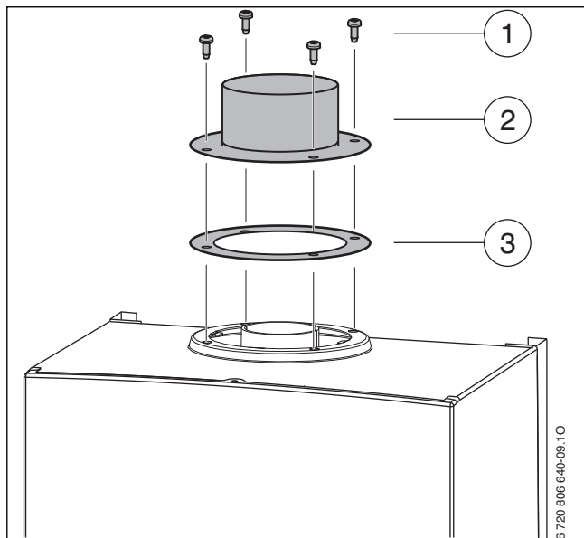
Рис. 18 Крепление переходника
