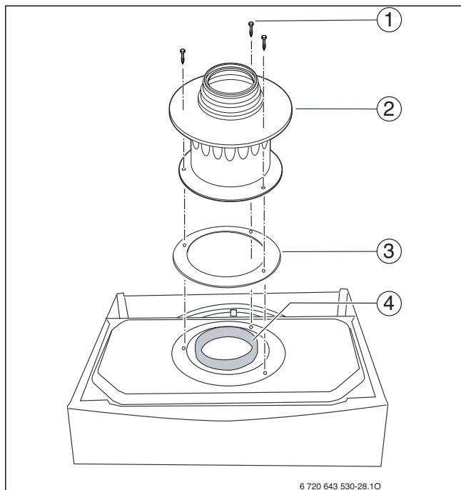
Рис. 19 Установка переходника дымовых газов В 22 и дроссельной диафрагмы
