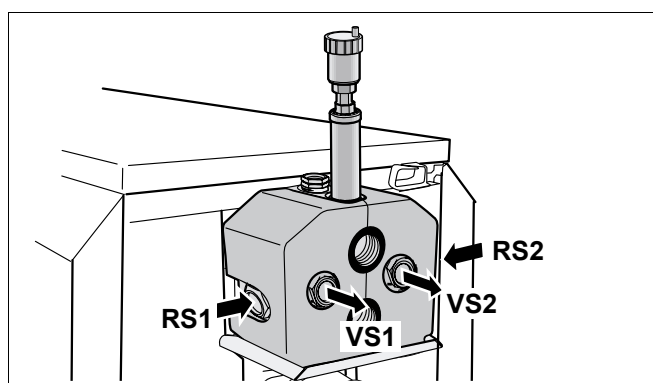
Рис. 54 Подключение бака-водонагревателя
