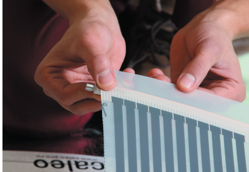
Рис. 8. Установленный на термопенку контактный зажим
