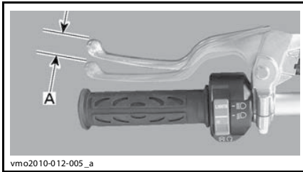
РЫЧАГ СЦЕПЛЕНИЯ - НОРМАЛЬНАЯ ВЕЛИЧИНА СВОБОДНОГО ХОДА A. 10 мм – 15 мм
