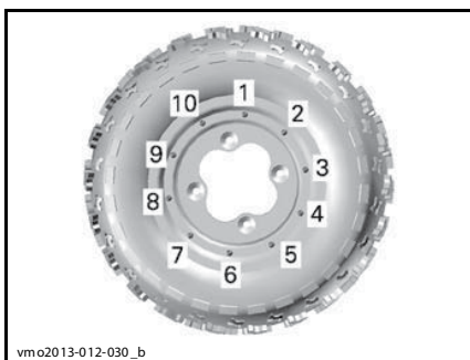
КОЛЕСА, ОСНАЩЕННЫЕ БЕДЛОКОМ С 10 БОЛТАМИ - ПОСЛЕДОВАТЕЛЬНОСТЬ ЗАТЯЖКИ (ИТОГОВЫЙ ШАГ)
