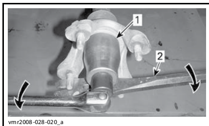
1. Торцевая головка на 41 мм 2. Лом
