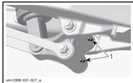
КОЛЕНЧАТЫЙ РЫЧАГ
