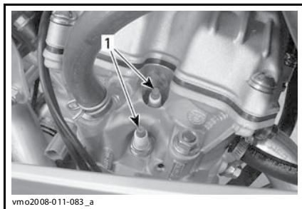
1. Свечи зажигания
