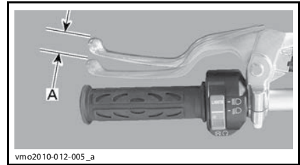
РЫЧАГ СЦЕПЛЕНИЯ - ПРАВИЛЬНАЯ РЕГУЛИРОВКА A. 10 мм – 15 мм
