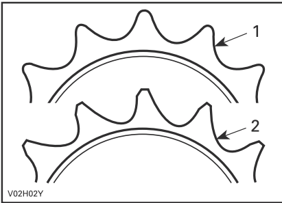
1. Исправное состояние 2. Требуется замена
