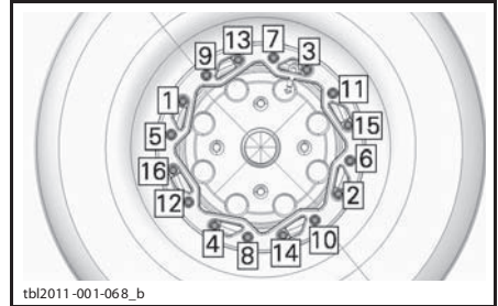
ТИПОВОЙ ВАРИАНТ — ПОСЛЕДОВАТЕЛЬНОСТЬ ЗАТЯЖКИ
