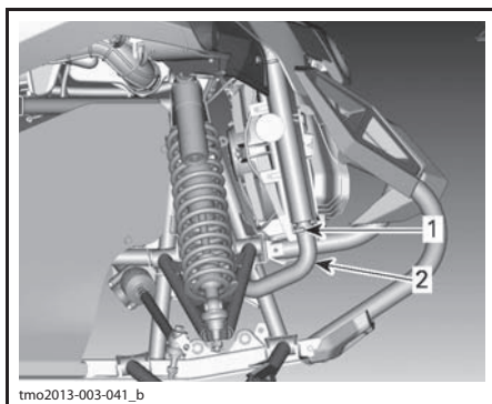
1. Запомните расположение хомута шланга 2. Снимите нижний шланг радиатора
