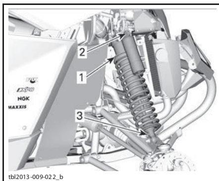
ПЕРЕДНЯЯ ПОДВЕСКА — МОДЕЛИ X rs
