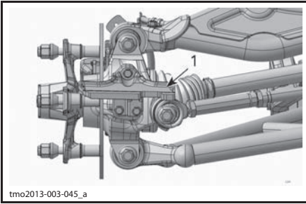
ДЛЯ НАГЛЯДНОСТИ КОЛЕСО СНЯТО 1. Колёсный скребок
