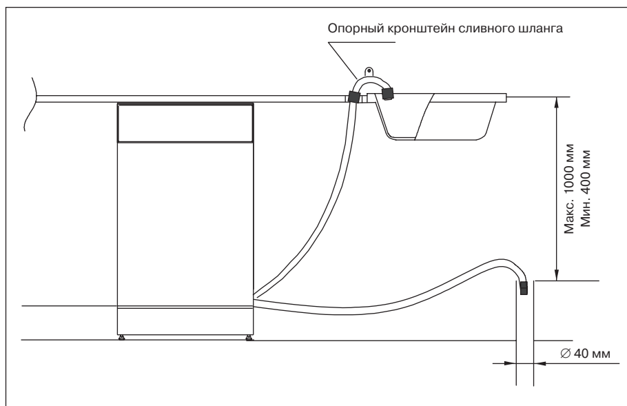
Рис. 6. Подключение слива.
