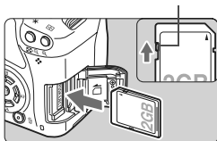
Переключатель защиты карты от записи
