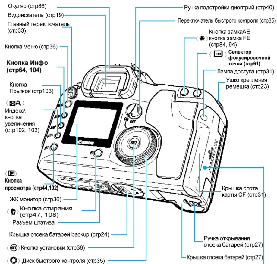
Вид под крышкой слота карты CF
