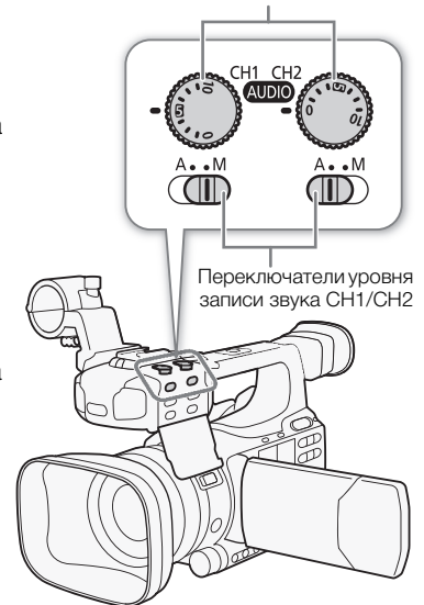
Диски уровня записи звука CH1/CH2
