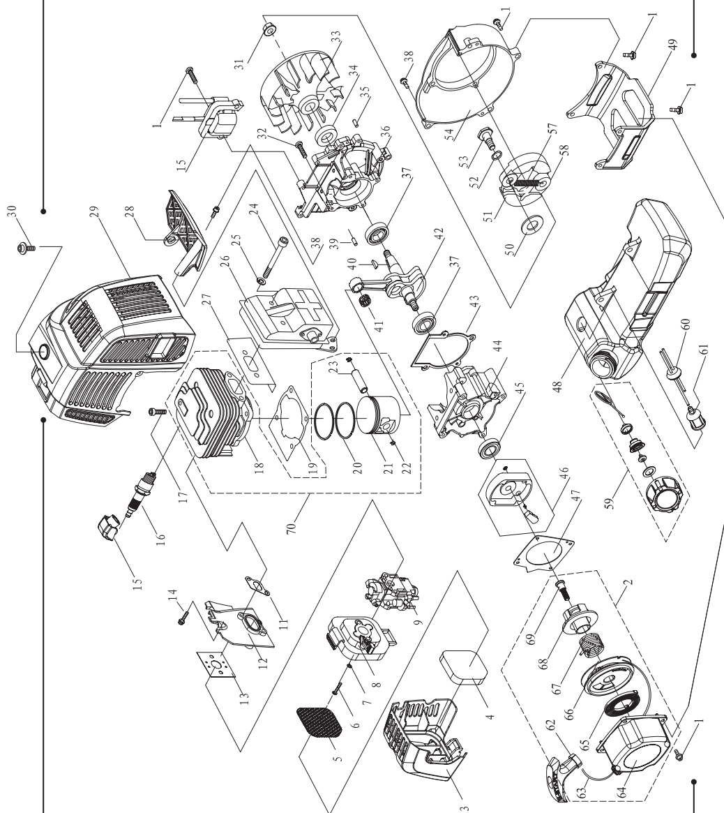
Рис. 18. Двигатель
