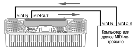
Контактное гнездо «MIDI IN» [Вход для сигналов MIDI] Контактное гнездо «MIDI OUT» [Выход для сигналов MIDI]
