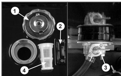
Рис. 7 Основные элементы топливного бака
