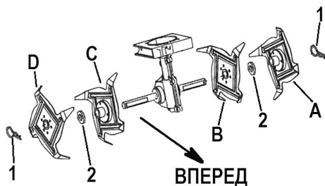
Рис. 4 Установка фрез
