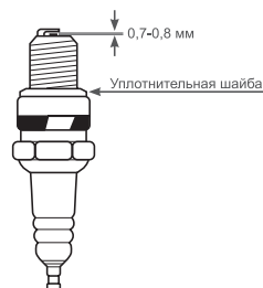
Рис. 13 Зазор между электродами свечи зажигания
