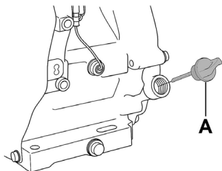
Рис. 6 Крышка-щуп маслозаливной горловины
