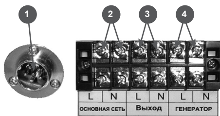
Рис. 14 Панель подключения блока ATS
