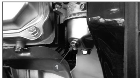
Рис. 21 Слив топлива из карбюратора 1. Болт сливной
