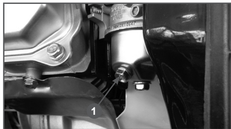
Рис. 16 Слив топлива из карбюратора 1. Болт сливной
