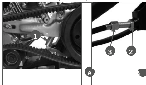
Рис. 6 Регулировка троса сцепления
