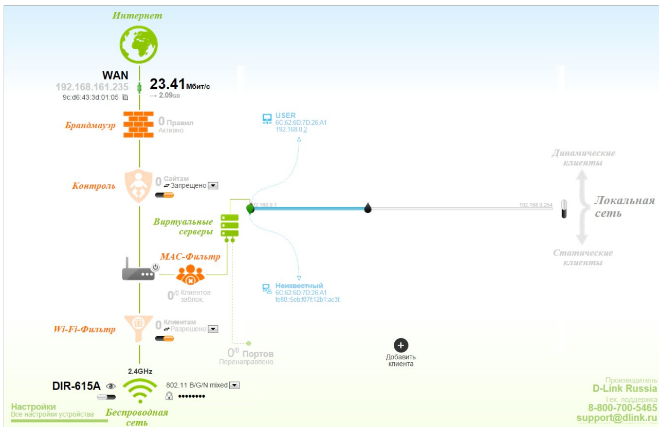
Рисунок 22. Страница Мониторинг.
