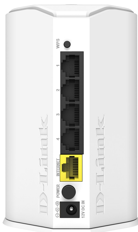
Рисунок 2. Вид задней панели DIR-615A.
