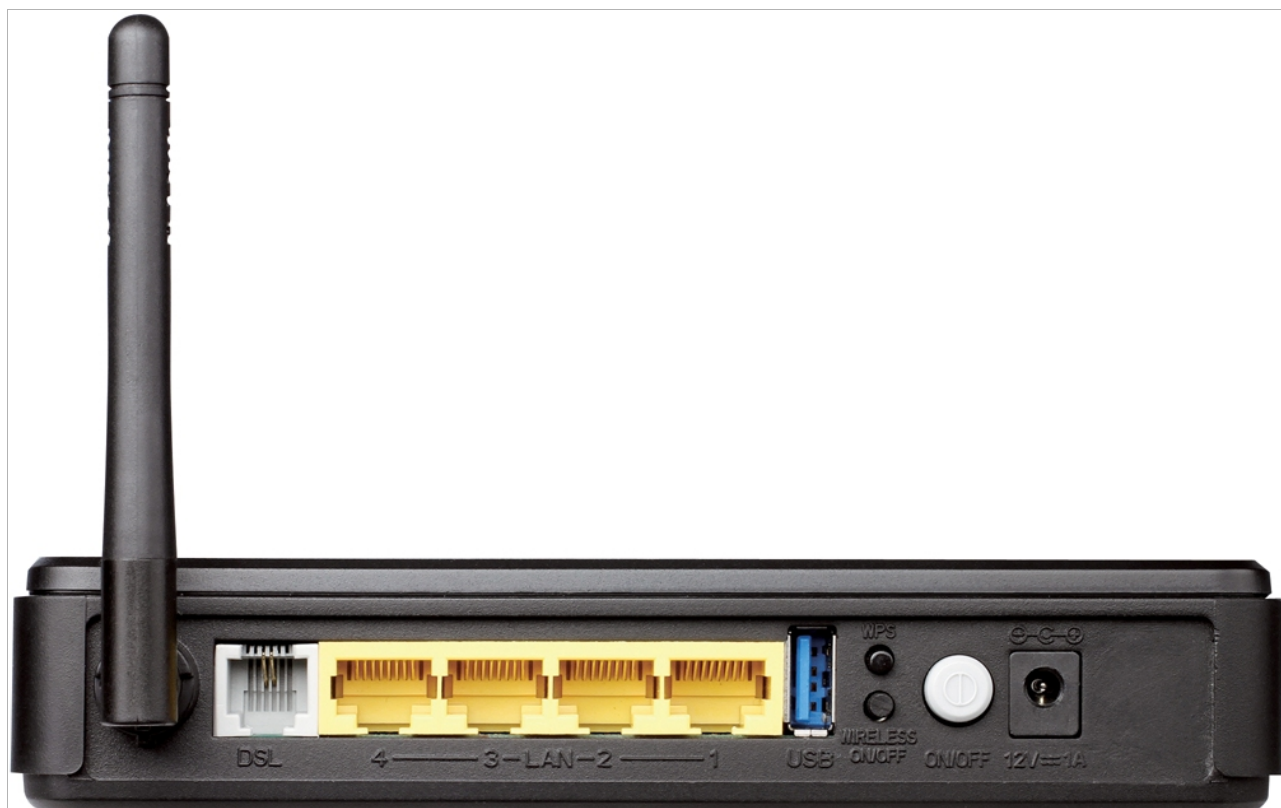
Рисунок 2. Вид задней панели DSL-2650U/NRU.
