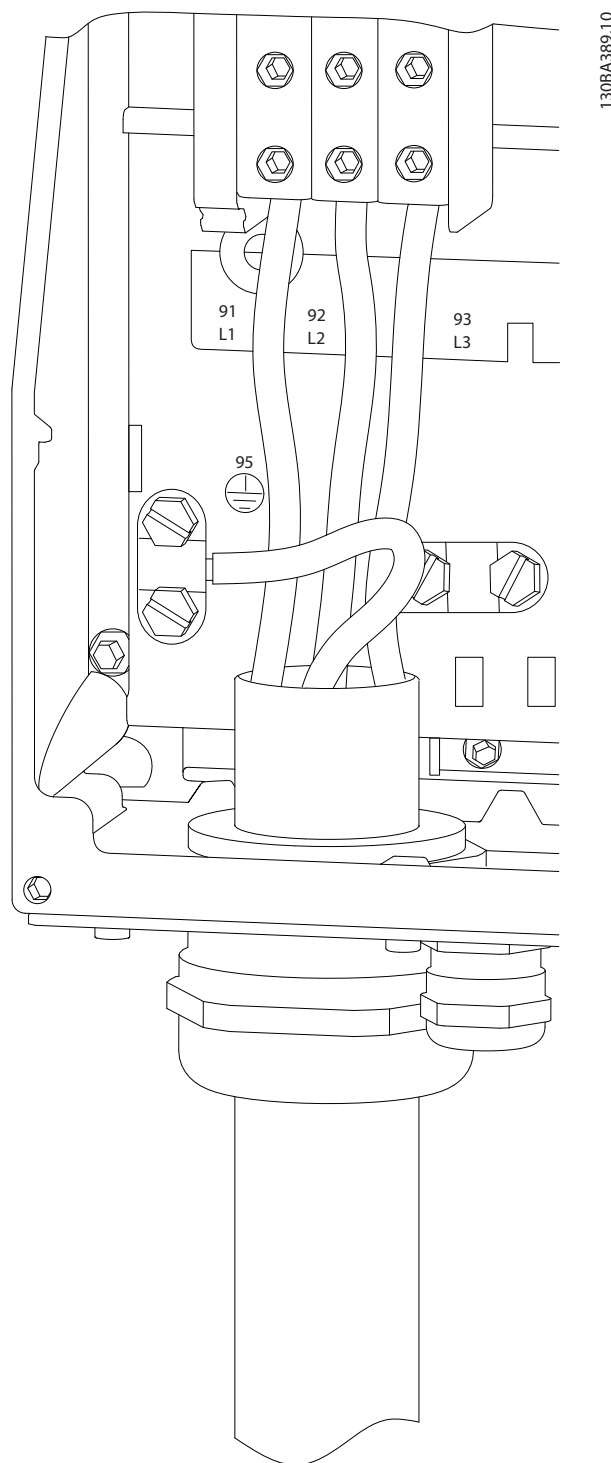
Рисунок 2.26 Подключение к сети и заземление, корпуса C1 и C2
