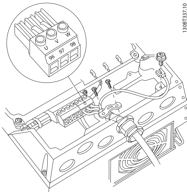
Рисунок 2.15 Подключение двигателя, корпуса A4 и A5
