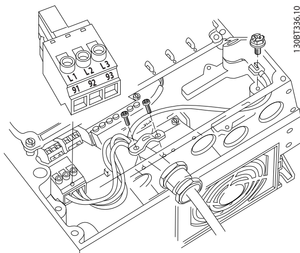
Рисунок 2.23 Подключение к питающей сети и заземлению без использования сетевого разъединителя
