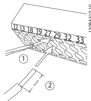
Рисунок 2.29 Подключение элементов управления
