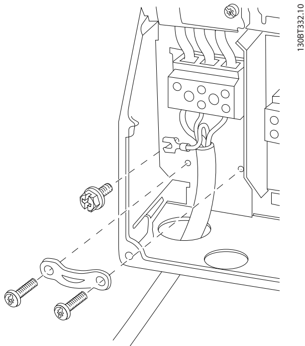
Рисунок 2.25 Подключение к сети и заземление, корпуса B1 и B2
