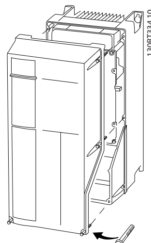
Рисунок 2.9 Доступ к подключениям проводки управления в корпусах A4, A5, B1, B2, C1 и C2
