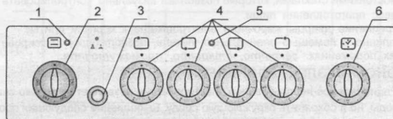
Панель управления плиты модели 506004.04э
