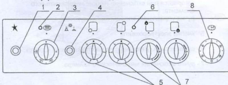
Панель управления плиты модели 5422.00гз
