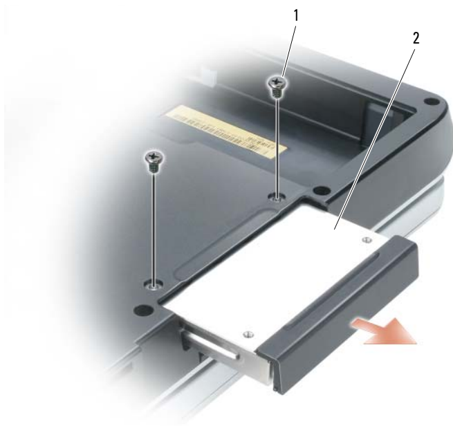
1 винты (2) 2 жесткий диск
