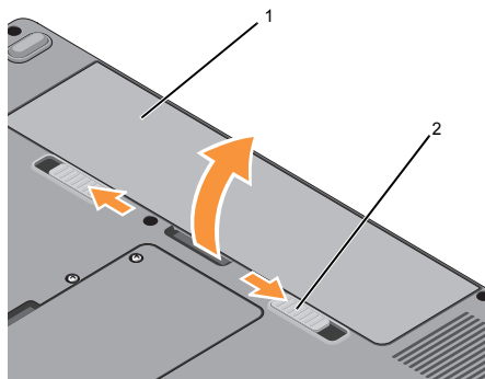
1 аккумулятор 2 фиксирующие защелки аккумуляторного отсека (2)
