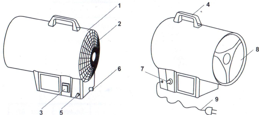
Рис.1. Устройство прибора
