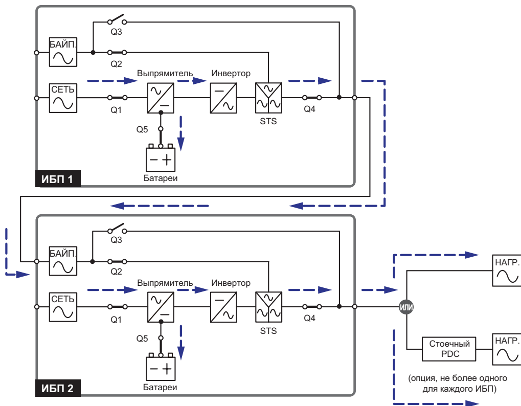
Рис. 3-10. Последовательное резервирование
