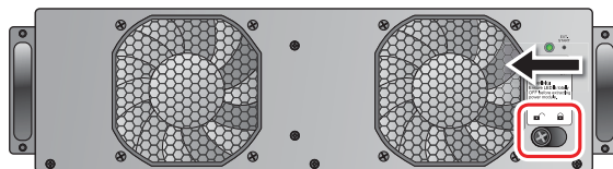
Рис. 5-23. Разблокировка защёлки
