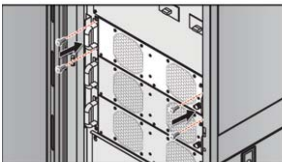
Рис. 5-21. Фиксация винтами
