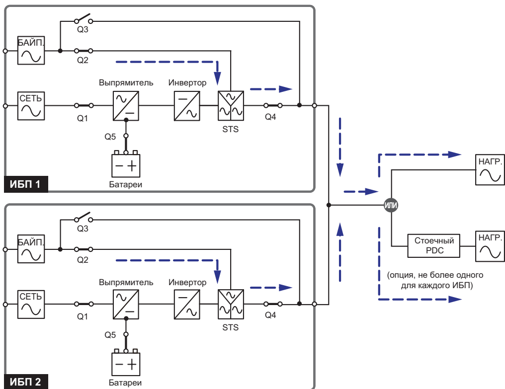
Рис. 3-8. Режим байпаса, система с несколькими параллельными ИБП
