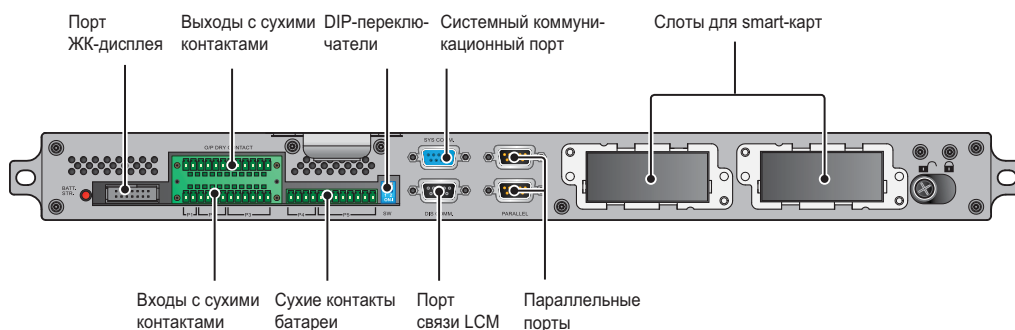
Рис. 4-2. Коммуникационные интерфейсы
