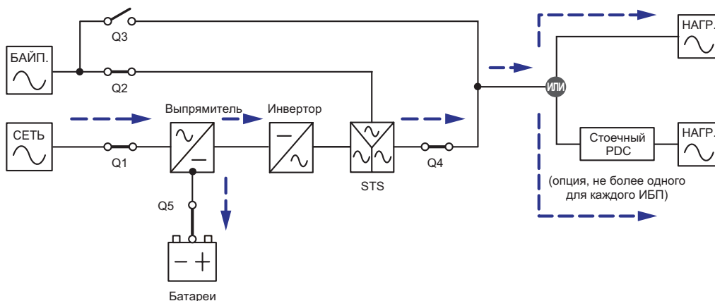
Рис. 3-1. Нормальный режим работы, система с одним ИБП
