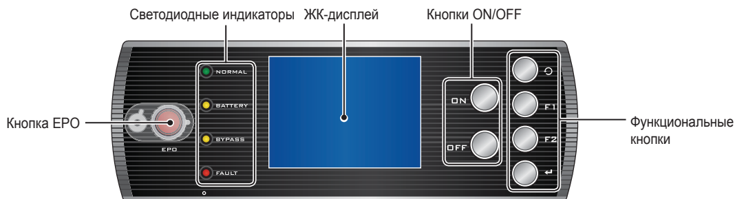
Рис. 2-8. Панель управления
