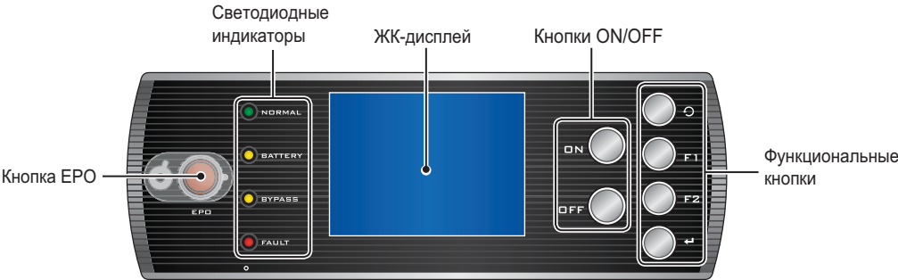
Рис. 7-2. Панель управления
