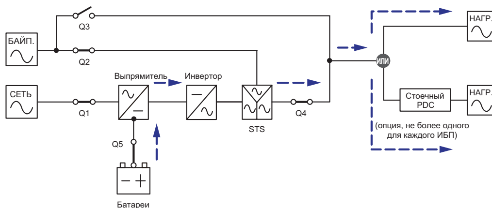
Рис. 3-2. Нормальный режим работы, система с одним ИБП
