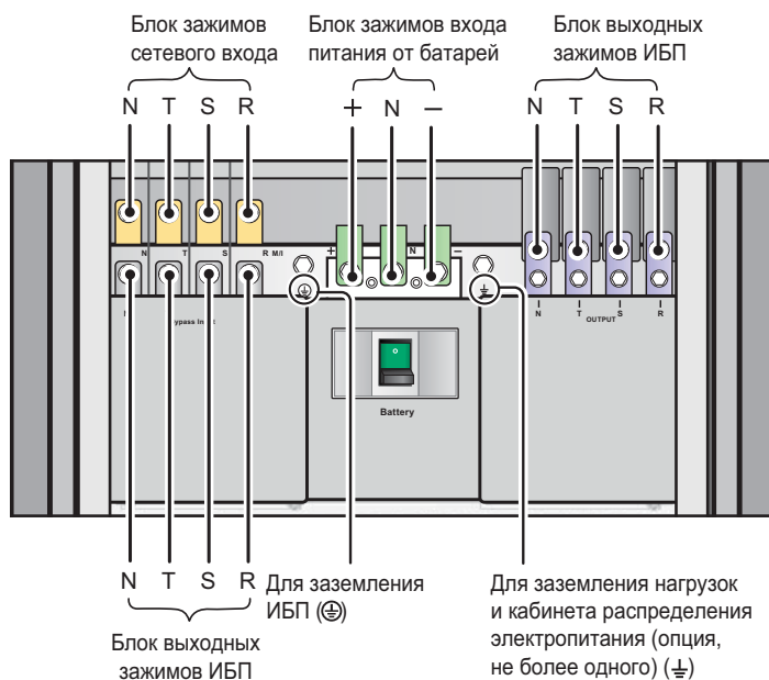
Рис. 5-8. Схема подключения в конфигурации с двумя входами (одиночный ИБП)
