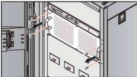
Рис. 5-29. Выкручивание винтов
