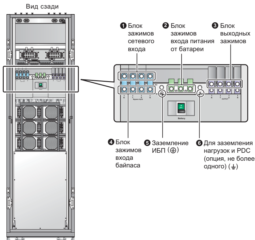
Рис. 2-10. Вид сзади: выходы ИБП
