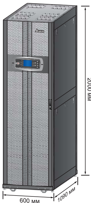
Рис. 2-2. Размеры
