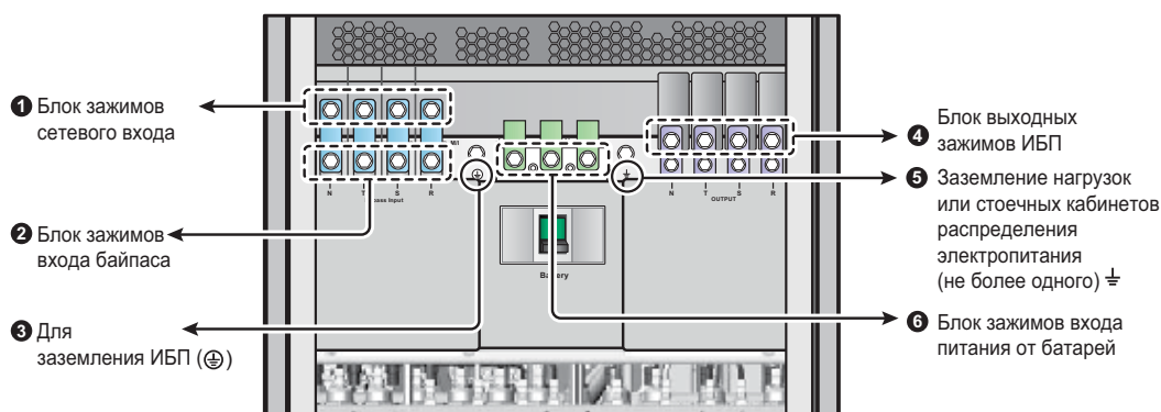
Рис. 5-5. Выводы ИБП
