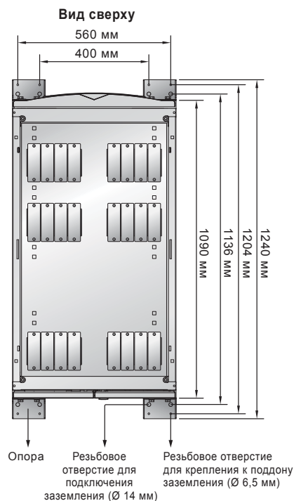
Рис. 2-3. Расположение крепежных отверстий
