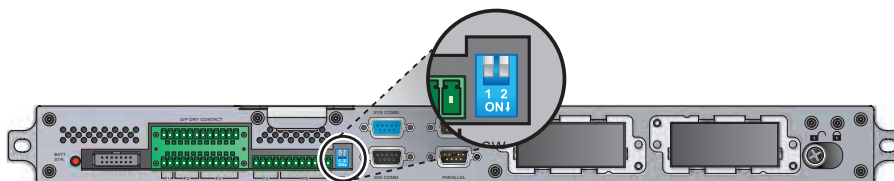
Рис. 6-2. DIP-переключатели
