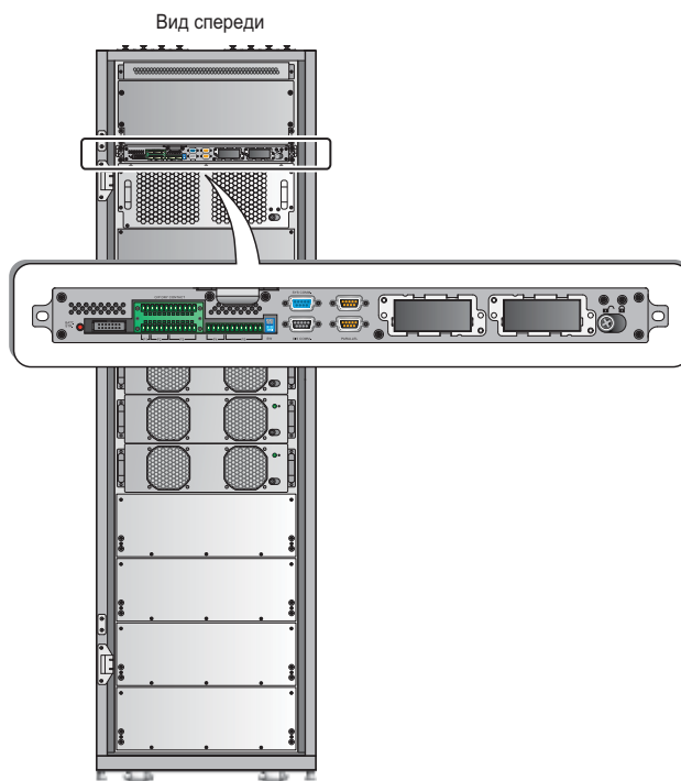
Рис. 4-1. Вид спереди: коммуникационные интерфейсы
