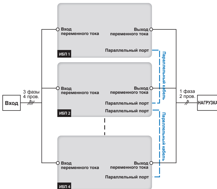
Рис. 6-17. Схема подключения в конфигурации с одним входом (система с параллельно включёнными ИБП)
