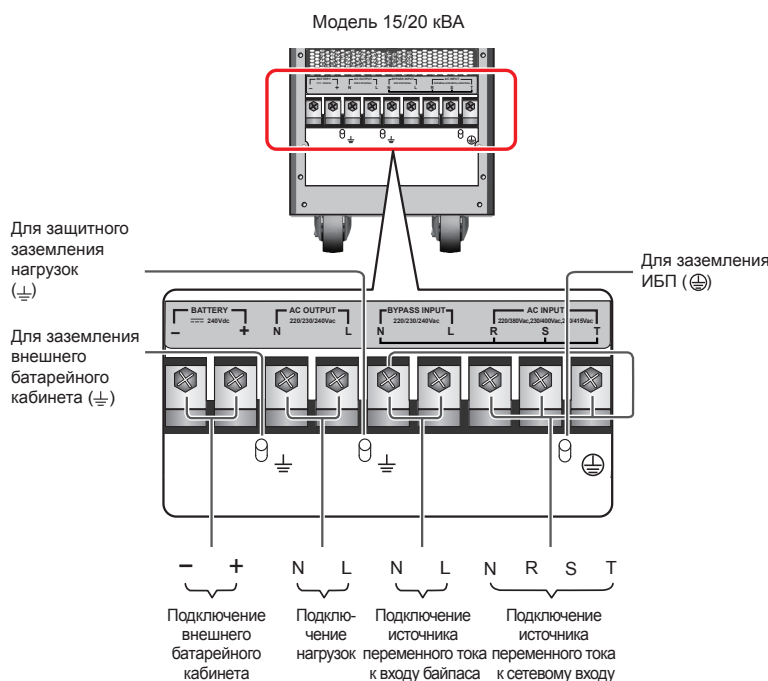
Рис. 6-16. Схема подключения одноконтурного ИБП 15/20 кВА в конфигурации с двумя входами
