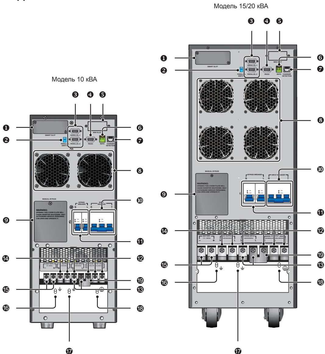
Рис. 3-3. Задняя панель
