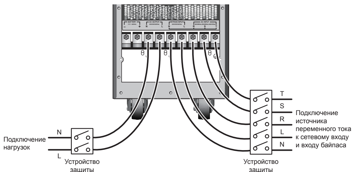
Рис. 6-9. Схема установки устройств защиты для ИБП с двумя входами
