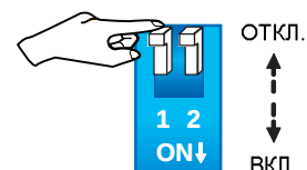
Рис. 5-2. Переключатель параллели
