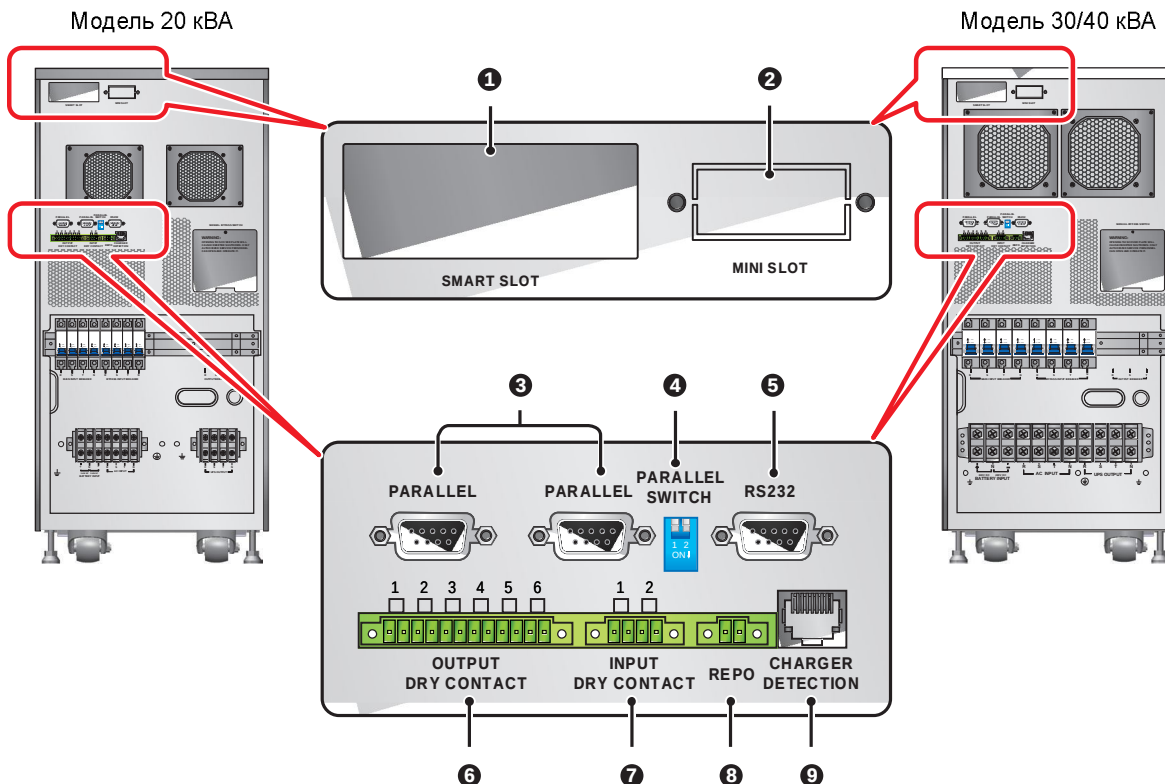
Рис. 5-1. Коммуникационные интерфейсы
