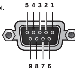
Рис. 5-3. Порт RS232
