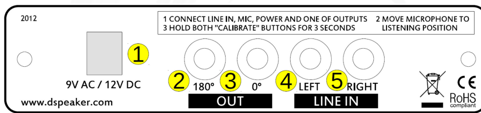
Задняя панель Anti-Mode 8033S-II
