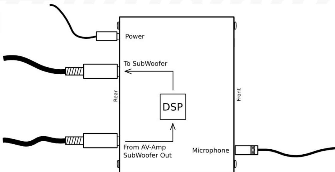
Схема подключения Anti-Mode 8033
