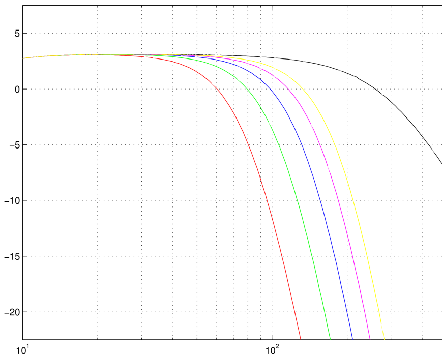
Anti-Mode 8033S-II ФНЧ
