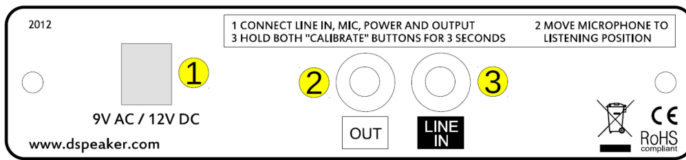
Задняя панель Anti-Mode 8033 cinema
