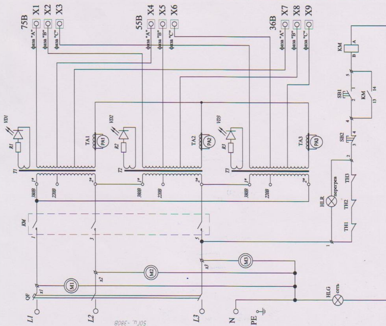
Рис.2. Схема электрическая принципиальная "Дуга СПБ-35"
