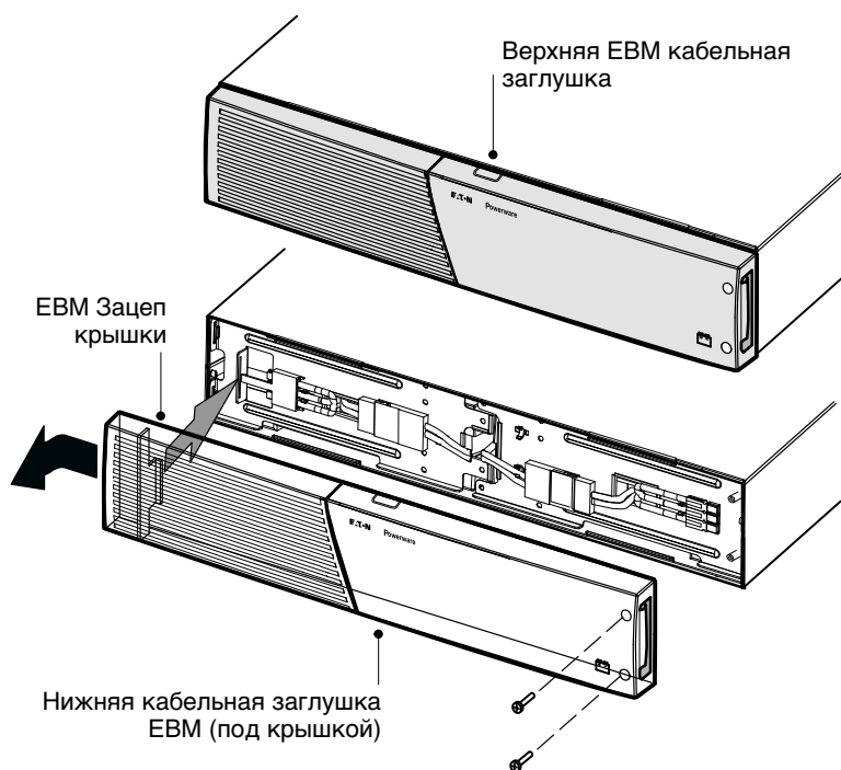
Рисунок 27. Снятие передней ЕВМ крышки
