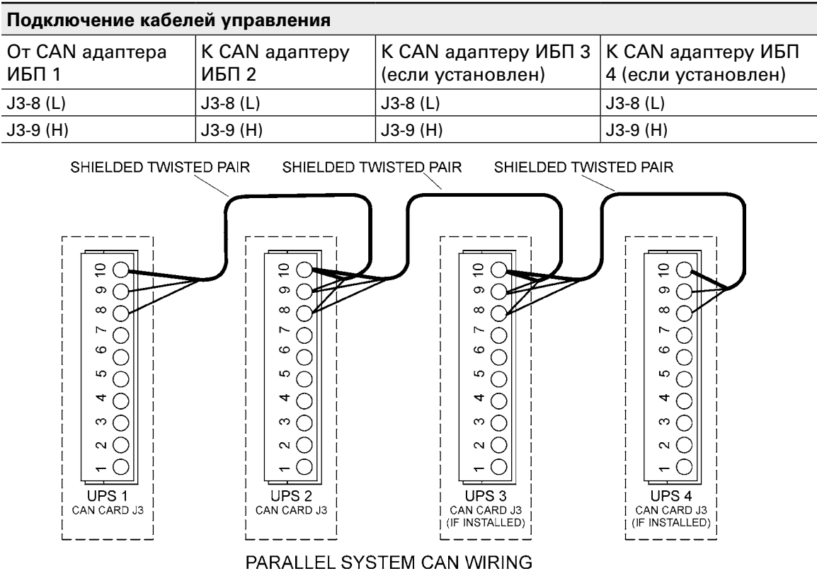
Рисунок 51. Монтаж информационных кабелей
