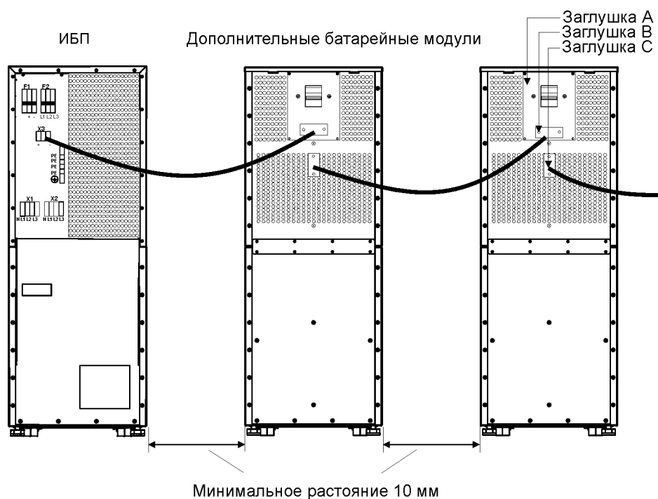
Рисунок 24. Схема соединения ИБП и батарейных модулей
