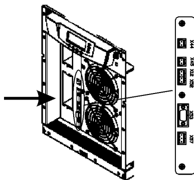
Рисунок 26. Расположение разъемов управляющего кабеля: сигнальные входы (X44 & X45); EPO (NC (X12) & NO (X52)); RS-232 (X53); релейный выход (X57)
