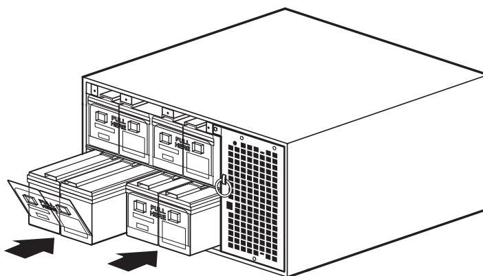
Рисунок 27. Установка аккумуляторных отсеков ИБП
