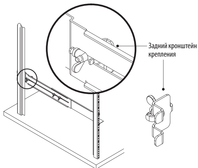
Рисунок 16. Закрепление задней части EBM
