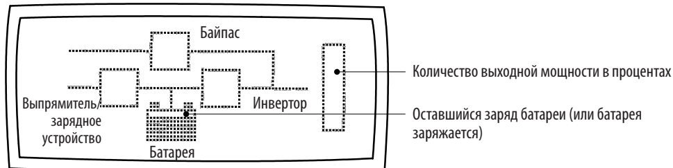
Рисунок 46. Окно "Mimic" модуля BladeUPS
