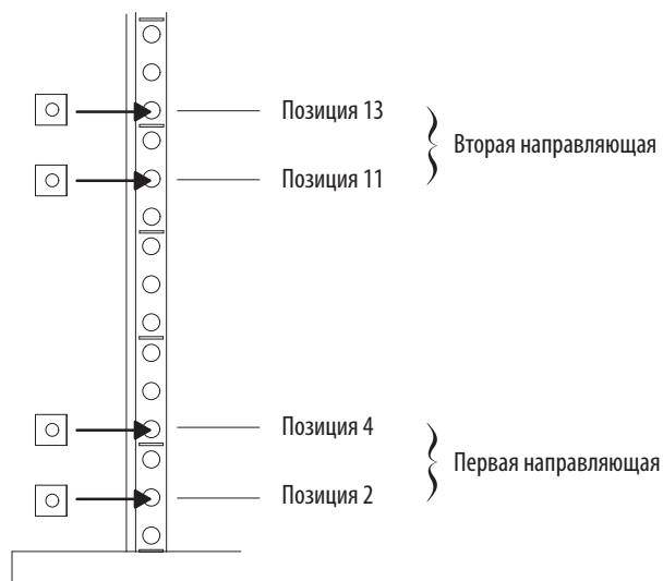
Рисунок 12. Положения винтов задней направляющей для ЕВМ
