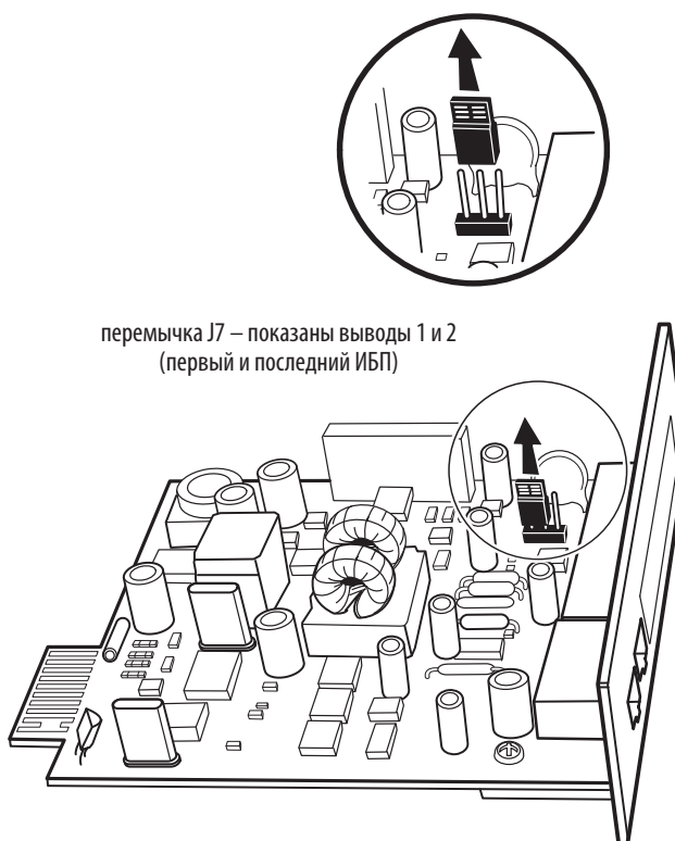
Рисунок 42. Извлечение перемычки J7 (вид сбоку)
