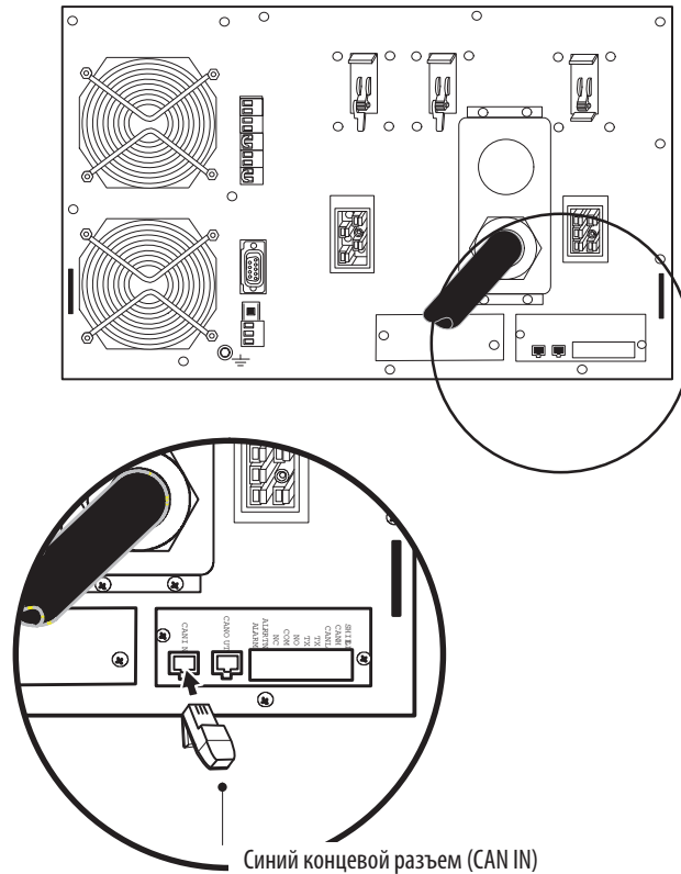
Рисунок 34. Установка синего концевой разъем (первый ИБП)
