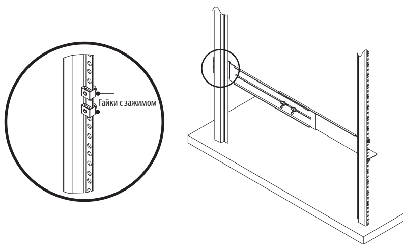
Рисунок 13. Закрепление задней направляющей
