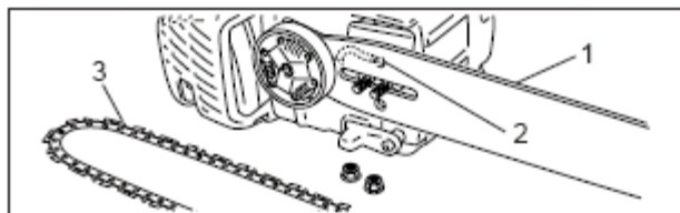
1. Желоб (канавки) пильной шины 3. Пильная цепь 2. Отверстие подачи масла
