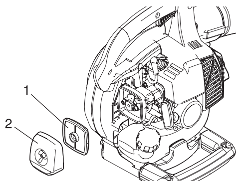
1. Воздушный фильтр
