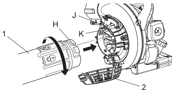
1. Всасывающая труба
