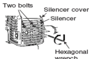
Крышка глушителя = Silencer cover; Глушитель = Silencer Два болта = Two bolts; Торцевой ключ = Hexagonal wrench
