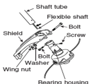
Трубка вала = Shaft tube; Винт = Screw Гибкий вал = Flexible shaft; Прокладка = Washer Крышка = Shield; Корпус подшипника = Bearing housing; Болт = Bolt
