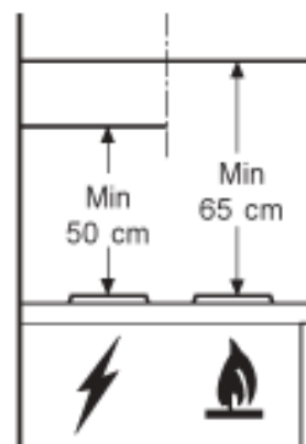
Рис. 6 - Установка
