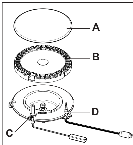
A - Cappellotto B - Spartifiamma C - Candeletta di accensione D - Termocoppia
