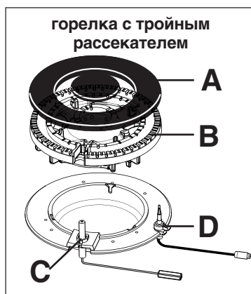
Рис. 2 A - Крышка B - Рассекатель горелки C - Свеча зажигания D - Термопара
