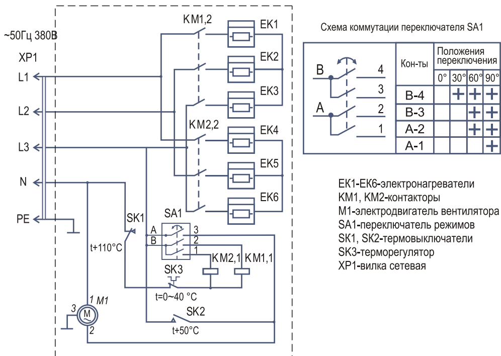
Рис. 2 Схема электрическая ТП12ЕТ, ТП18ЕТ
