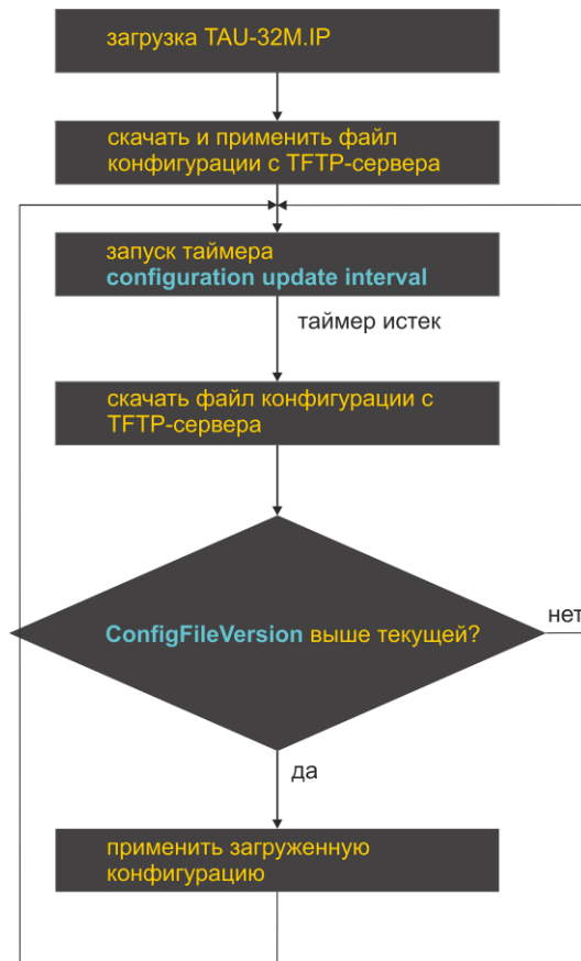
Рисунок 23 – Алгоритм работы функции автоматического конфигурирования TAU-32M.IP и проверки актуальности файла конфигурации
