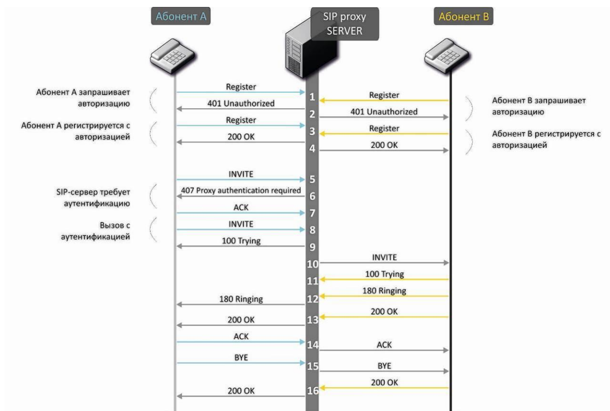
Рисунок 19 – Алгоритм вызова с участием SIP проху-сервера
