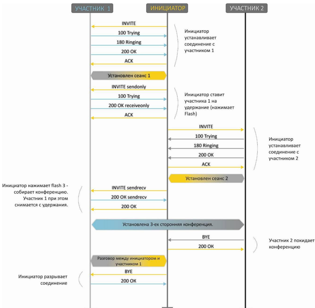
Рисунок 17 – Алгоритм выполнения услуги «3-way conference» по протоколу SIP
