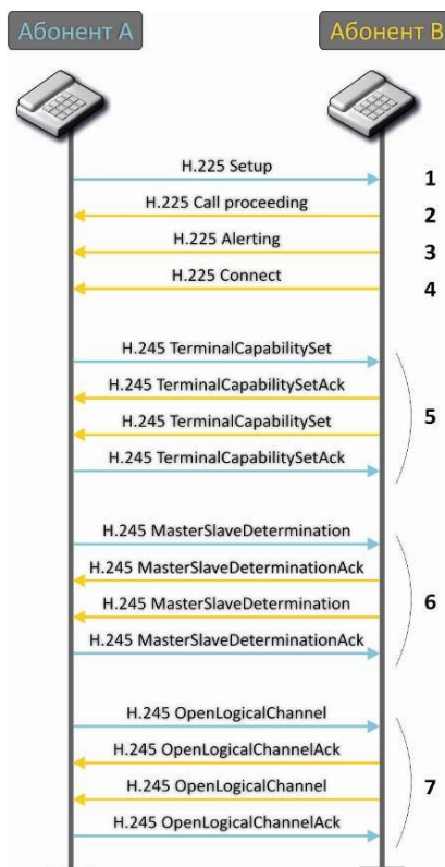
Рисунок 21 – Алгоритм вызова по протоколу H.323
