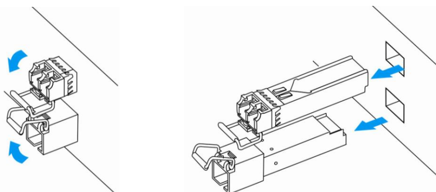
Рисунок 14 – Открытие защелки SFP-трансиверов и извлечение SFP-трансиверов
