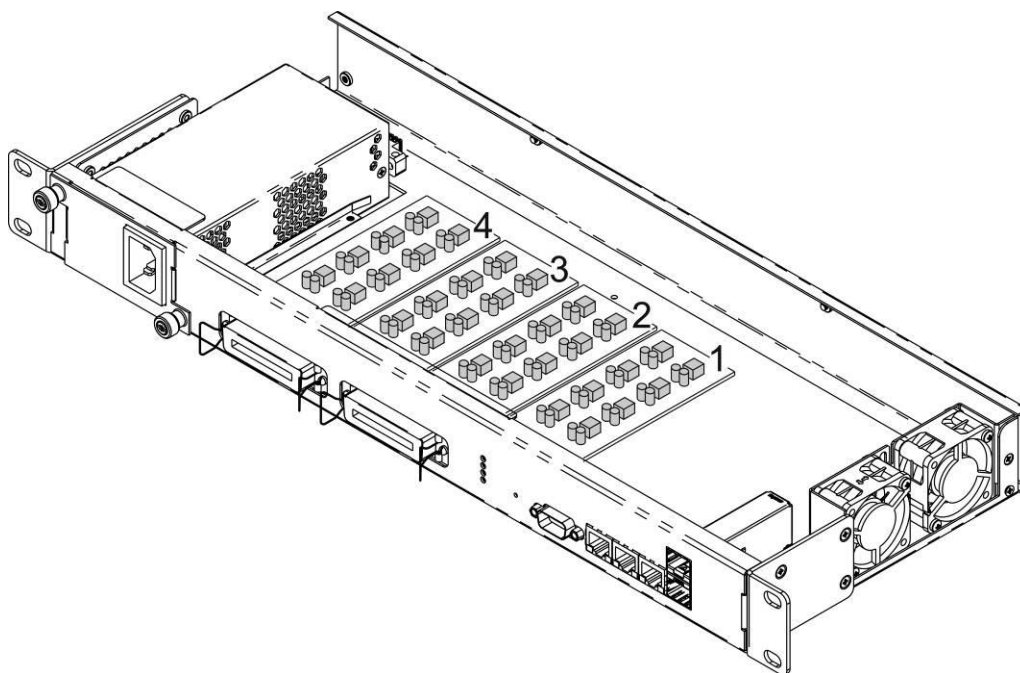
Рисунок 12 – Расположение submodule в TAU-32M.IP.
