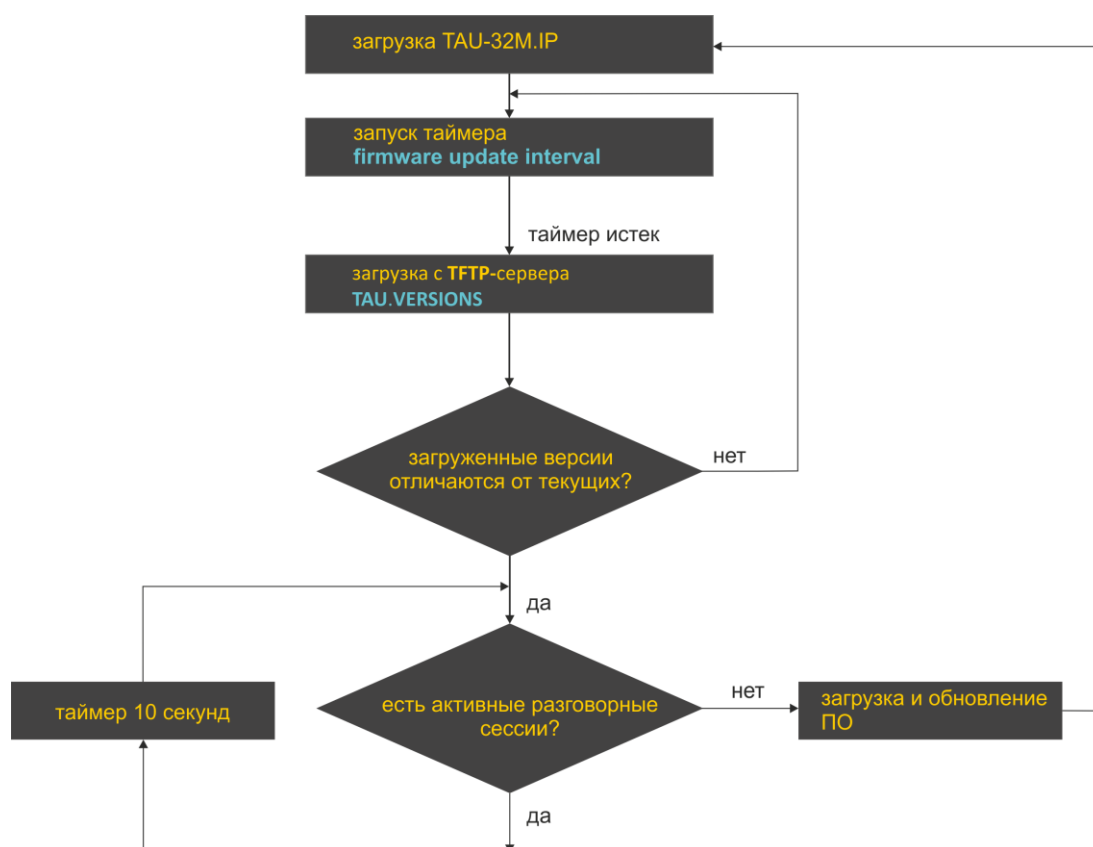
Рисунок 24 – Алгоритм работы функции автоматического обновления и проверки актуальности ПО
