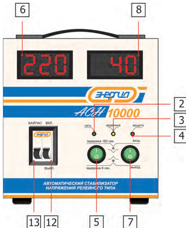
Лицевая панель
