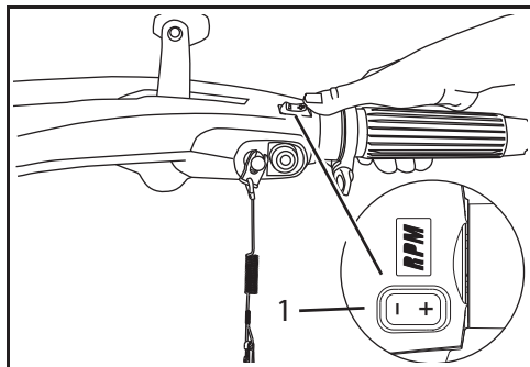
1. Переключатель Touch Trol 007068
