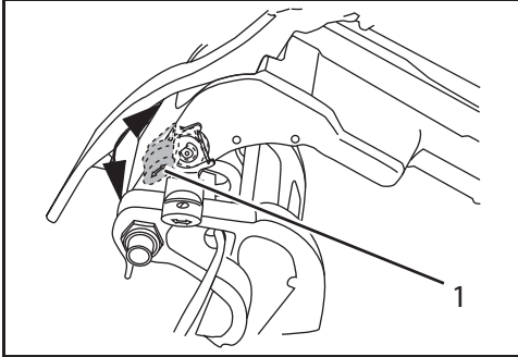
1. Рукоятка упора фиксации мотора в поднятом положении 007029
