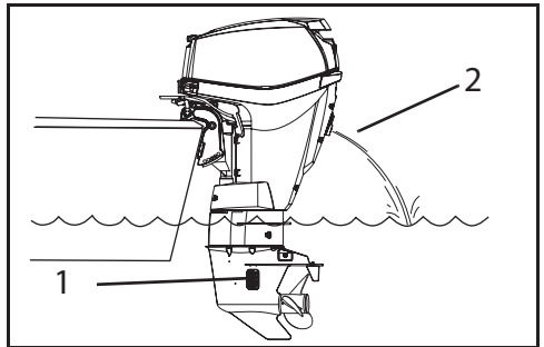
1. Отверстия водозабора 007031 2. Контрольное отверстие системы охлаждения
