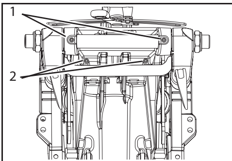
1. Втулка подъёма мотора (смазывать ежегодно) 007033 2. Вал рычага подъёма мотора (смазывать ежегодно)
