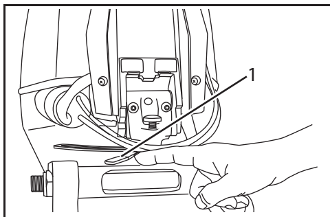
1. Рычаг регулировки усилия на руле 007042
