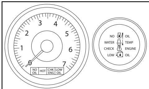
Типовой индикаторный прибор системы SystemCheck 008491
