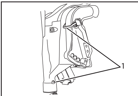
1. Точки смазки рычага и кронштейна для подъёма мотора (смазывать ежегодно) 007032
