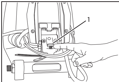
1. Регулировочный винт 007020
