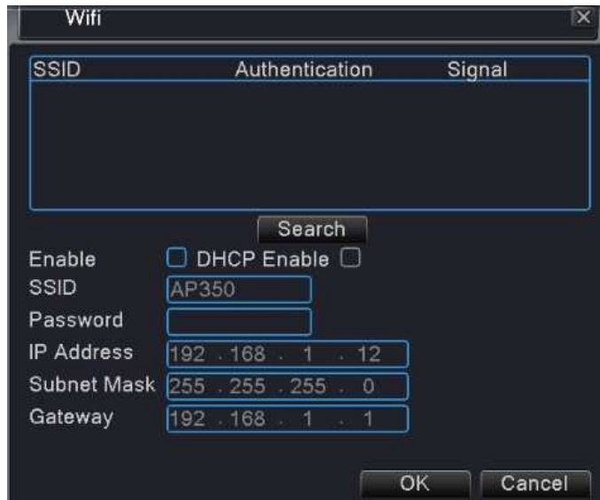
Рис. 4.28 Wi-Fi
