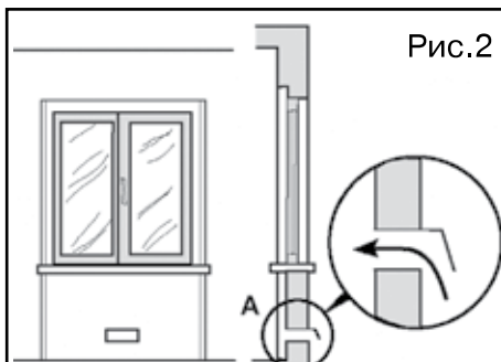
Пример обеспечения притока воздуха
