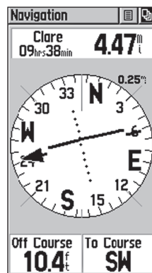
Навигационная страница с активным указателем курса и индикатором отклонения от курса (CDI). С помощью кнопок ZOOM Вы можете настроить шкалу CDI
