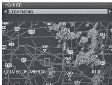
Рис.: Данные молнии.
