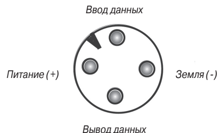
Внешний вид порта питания/данных прибора
